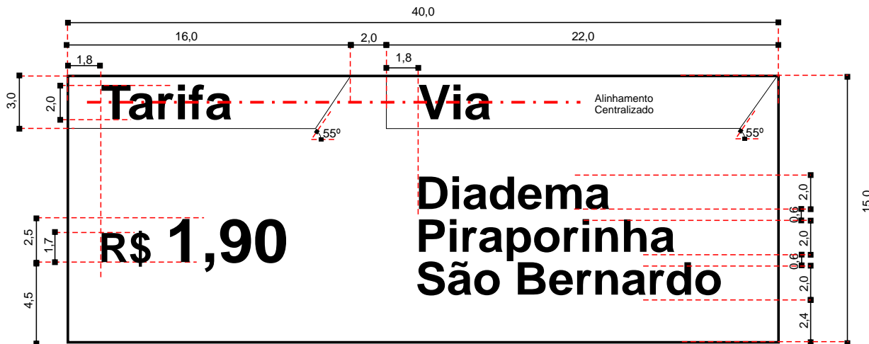
Placa de tarifa e itinerário - Diagramação
