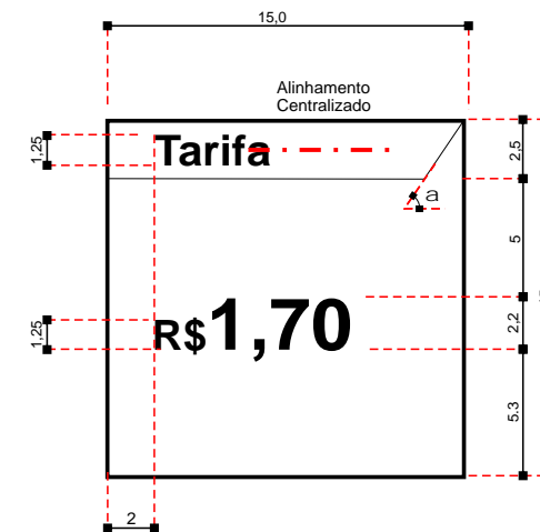
Placa tarifa - Diagramação
